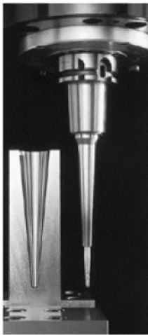
焼きばめホルダ 「スリムライン」
